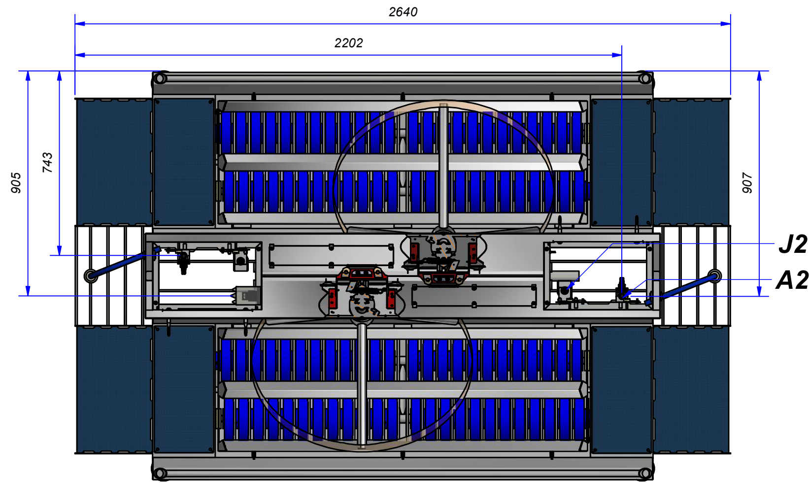
A-A (1:15)
